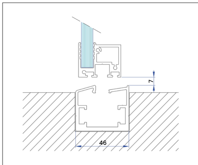
POSA INCASSATA CON BINARIO INFERIORE STANDARD
