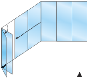
Configurazione con angolo 90° Tuttovetro; apertura SX singola interna pomo singolo
