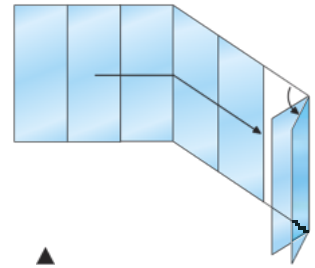
Configurazione con angolo 90° Tuttovetro; apertura DX singola interna pomo singolo
